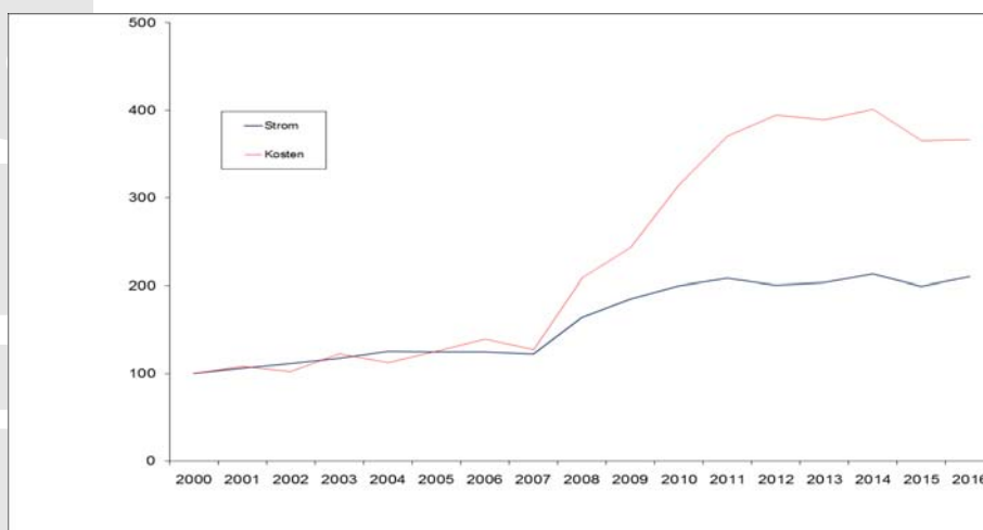
(100 für den Stromverbrauch entspricht 1.101,4 MWh, 100 für die Kosten entsprechen 96.9 T€)
